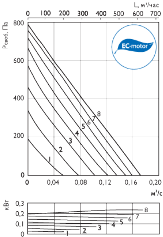
HERU 130 T EC приток
