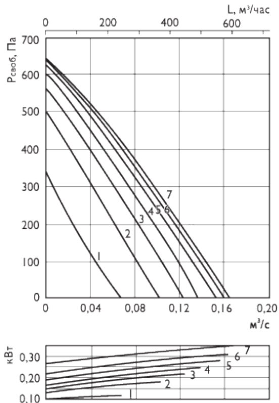
HERU 140 T приток
