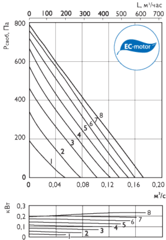
HERU 130 T EC вытяжка
