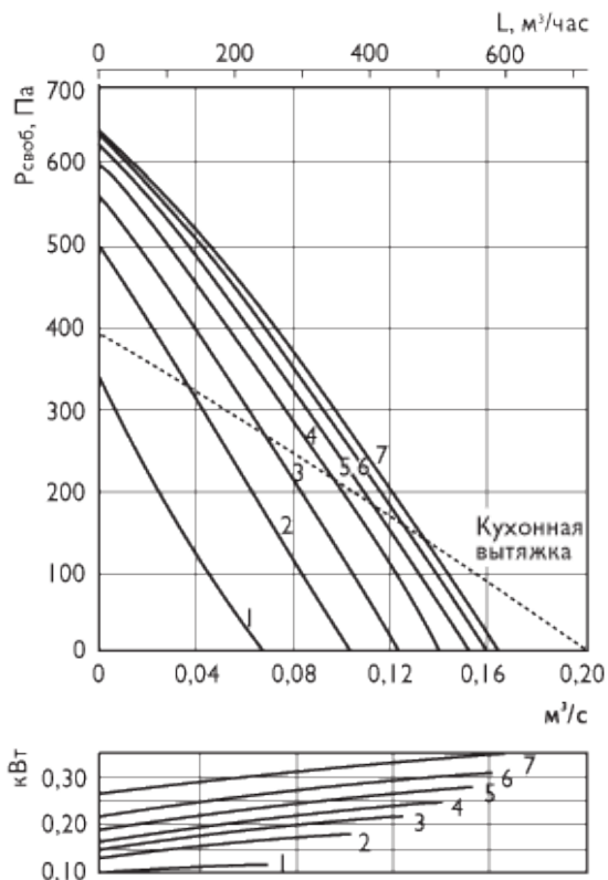
HERU 140 T вытяжка
