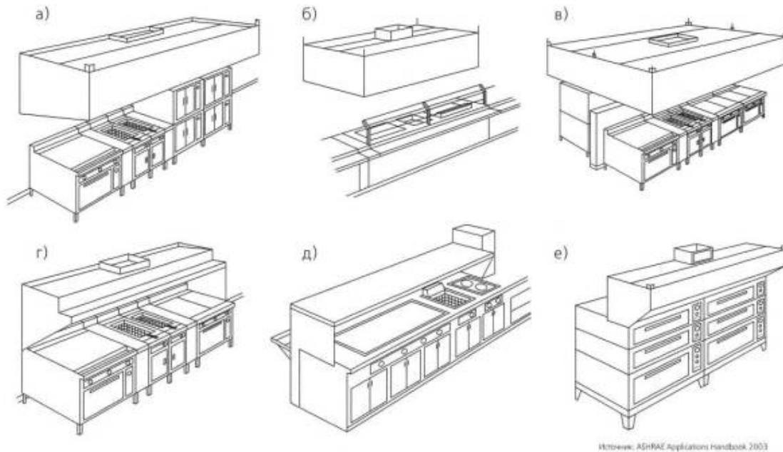
Рисунок 1 - Виды местных отсосов:
