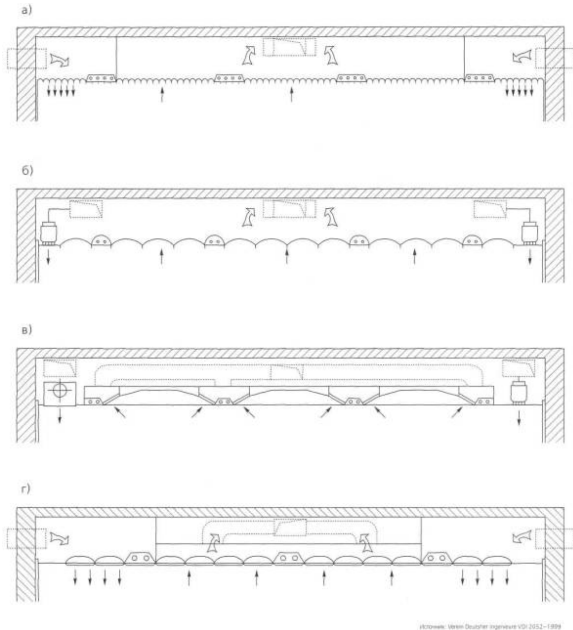
Рисунок 3 - Вентилируемые потолки:
